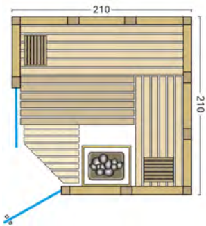
Abbildung Classico mit Sonderausstattung: Tür ohne Schwelle, 2 große Glaselemente, Dachschräge, LED-Beleuchtung, Inneneinrichtung Interio, VITALight-IPX4-Strahler mit Rückenpolster, Finnischer Saunaofen Eterno, Steuerung Saunacontrol T4.
